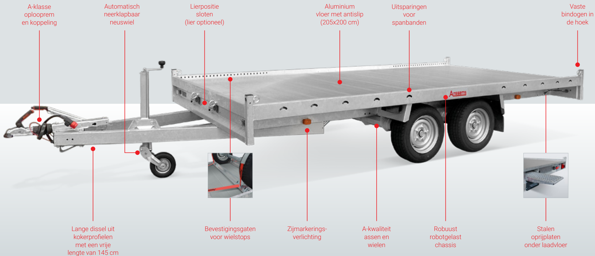
Aluminium laadvloer en bindogen in de hoeken
